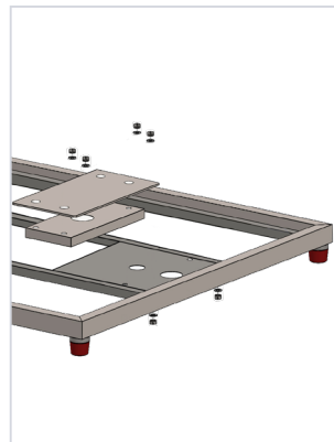
Y-K90031 Bodenplatte 80 × 80 cm, Edelstahl
